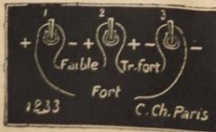
Fig. 1233-9. — Rôle des trois bornes 1, 2, 3 (fig. 8) prises deux par deux. Les pôles varient suivant la combinaison.
